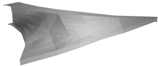
Finite-Element-Modell Twistträger
